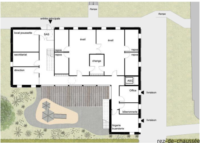
rez-de-chaussée
