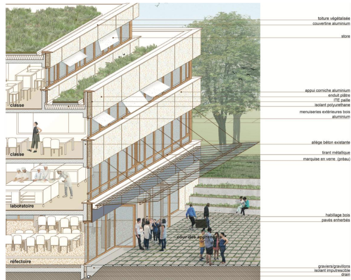
Rénovation de la façade du bâtiment CFA
