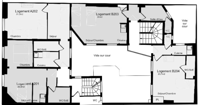
deuxième étage
