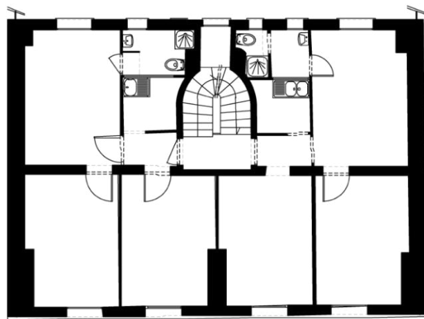
2EME ÉTAGE
