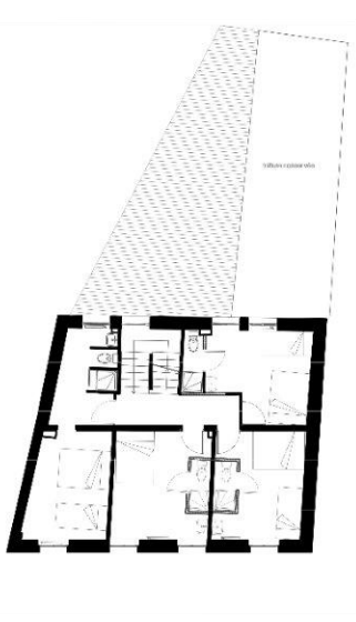
2, 3, 4eme étages
