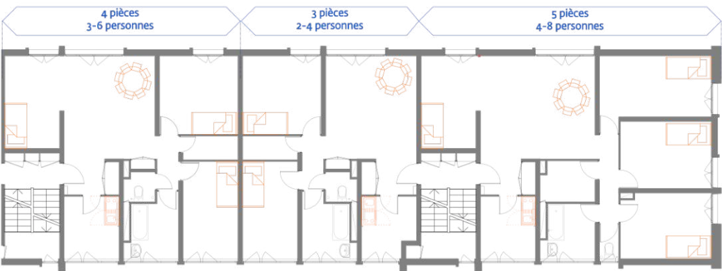
Plan d'aménagement logement par typologie
